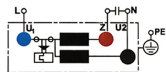
电气接线图
